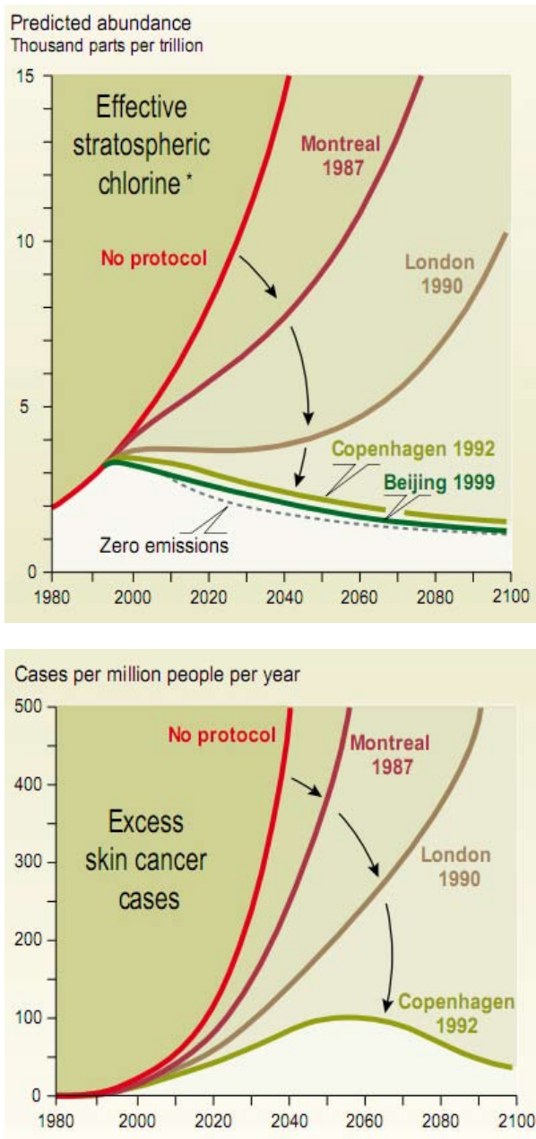
Figure 7. Effets du Protocole de Montréal et de ses amendements sur l'élimination des substances appauvrissant la couche d'Ozone (haut) et sur la fréquence des cancers de la peau (bas). http://www.grida.no/graphic.aspx?f=series/vg-ozone/08-Effects-of-the-Montreal-Protocol.jpg
