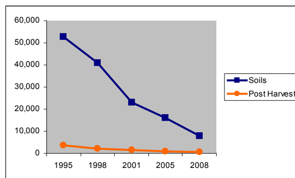
Figure 3. Evolution de la consommation du Bromure de Méthyle (désinfections des sols et post récolte) de 1995 à 2008 (TEAP Octobre 2008)
